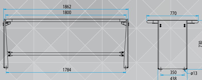
TAFELBLAD HARMONY DRAADRASTER – STEUNPOTEN QUADRI MAXI MOBIEL
