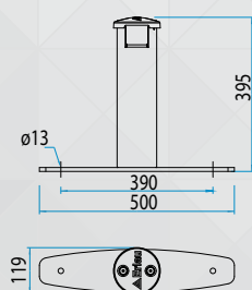
STEUNPOOT VARI MOBIEL / MET BEVESTIGINGSGATEN
