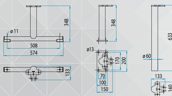
STEUNPOOT NOVA ENKEL MOBIEL / FPO / VAST IN BETON FUNDERING
