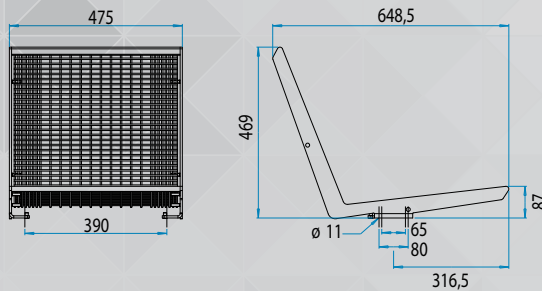
TOPSIT PAGHOLZ MET RUGLEUNING
