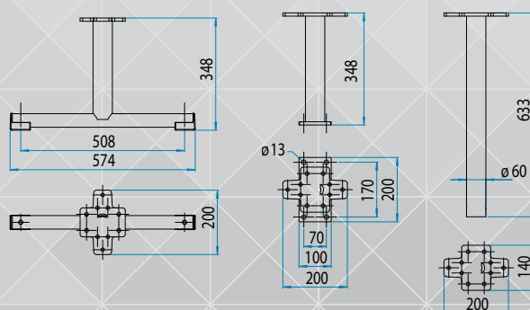
STEUNPOOT NOVA DUBBEL MOBIEL / FPO / VAST IN BETON FUNDERING
