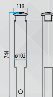
STEUNPOOT NOVA ENKEL MOBIEL / FPO / VAST IN BETON FUNDERING
