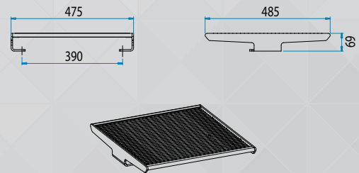
TOPSIT DRAADRASTER ZONDER RUGLEUNING
