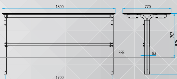
TAFELBLAD STYLE – STEUNPOTEN TABULA VAST
