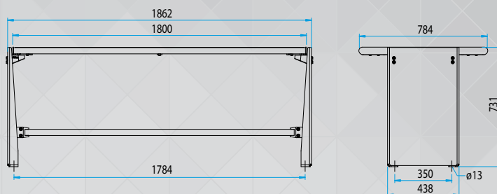
TAFELBLAD STYLE – STEUNPOTEN QUADRI MAXI MOBIEL
